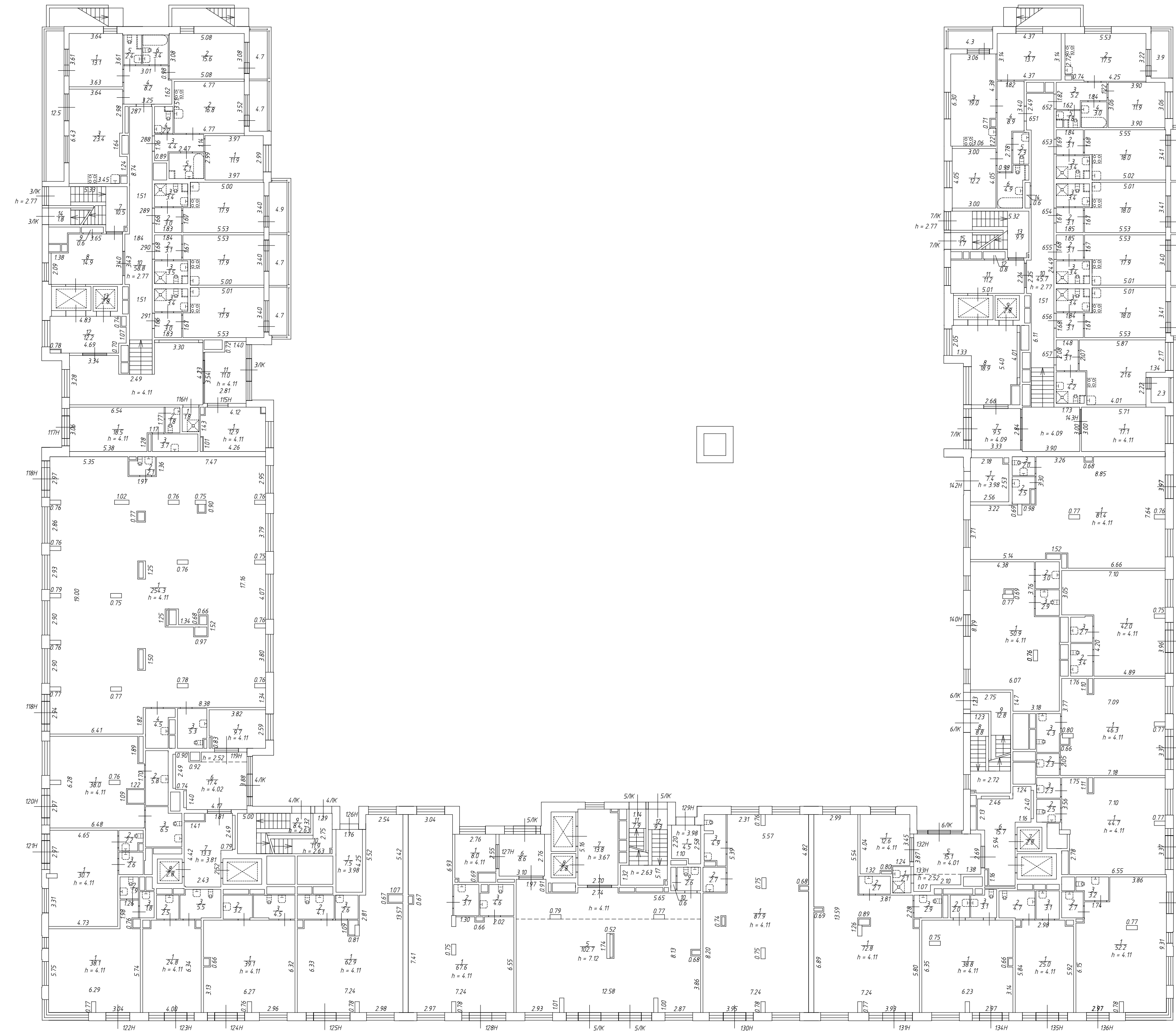
План 1 этажа
